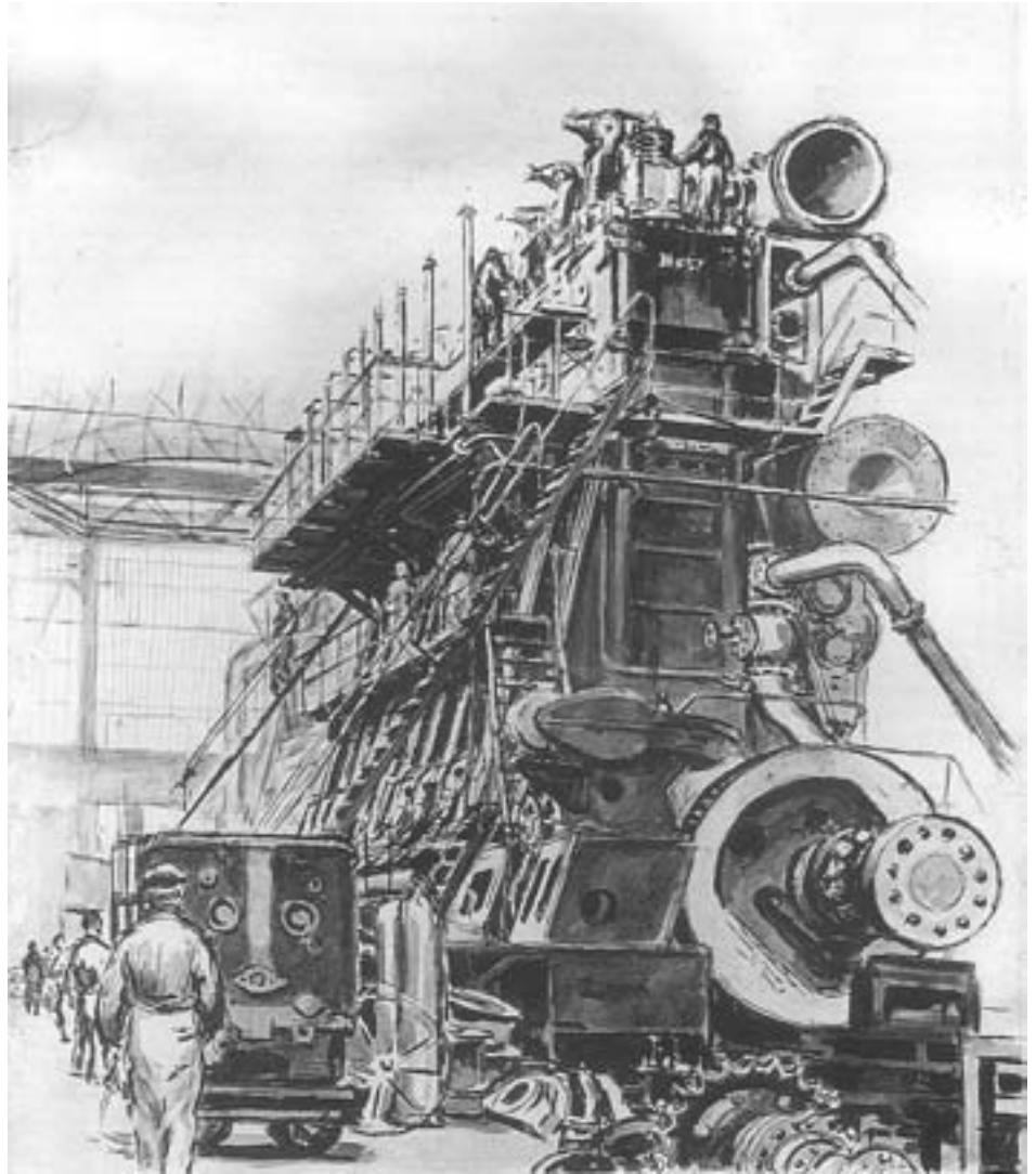
B&W. Den store dieselmotor bygges Tegning, blyant og tusch. 1952
